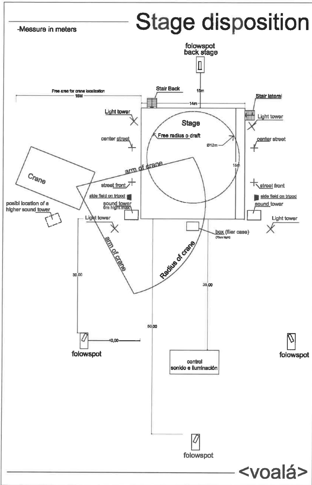
II. 3. Rozmieszczenie dźwigu (crane) względem sceny (stage) i obszaru realizacji wydarzenia.
